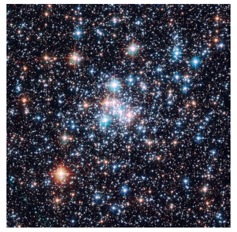
Star
