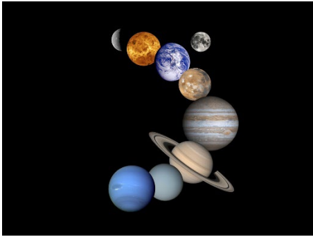
Planet
